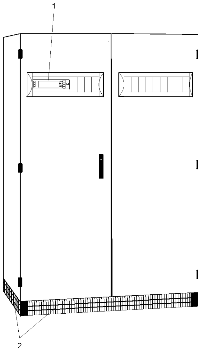
Bild 1 Beispielmodell 20 kVA (Bemaßungen siehe Kapitel 2, Tabelle 1)
