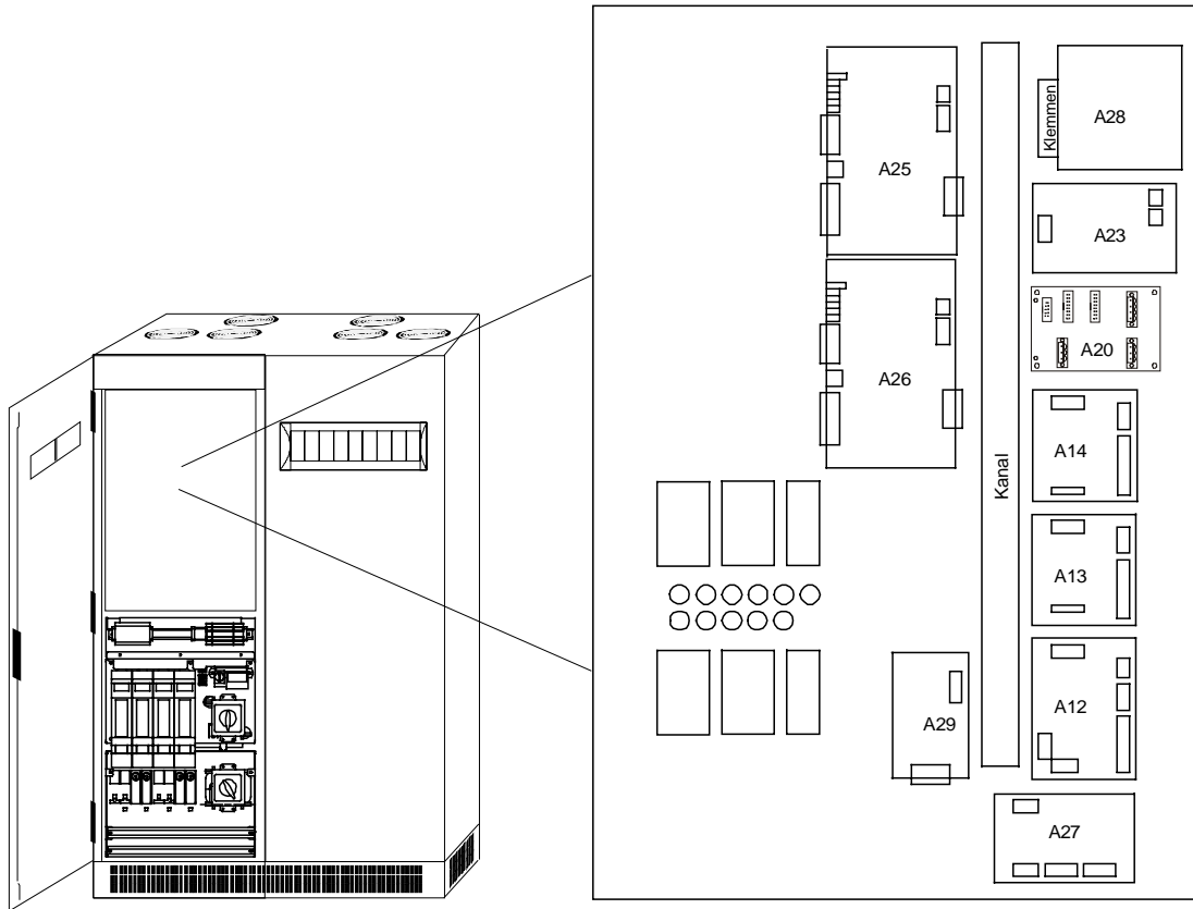
Bild 23 Leiterkarten auf dem Steuergeräteschwenkblech (Beispielmodell 40 kVA)
