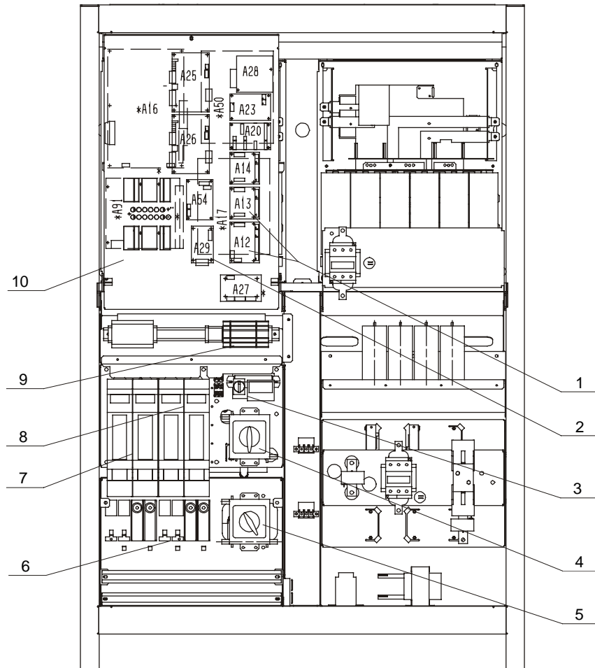
Bild 3 Anordnung der Bedien-, Bauelemente und einzelner Leiterkarten nach Öffnen der Türen (Beispielmodell 20 kVA).
