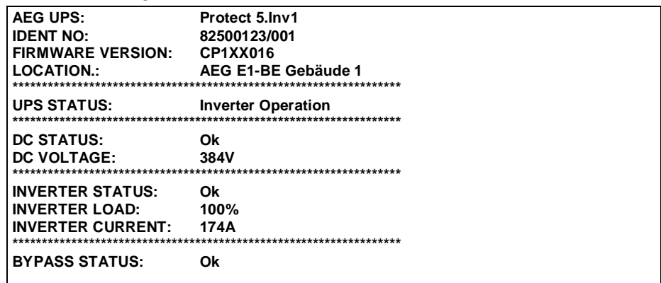
Bild 24 VT-100 Bildschirmaufbau
