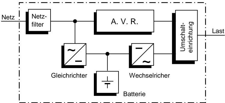
USV Blockschaltbild PROTECT A.
